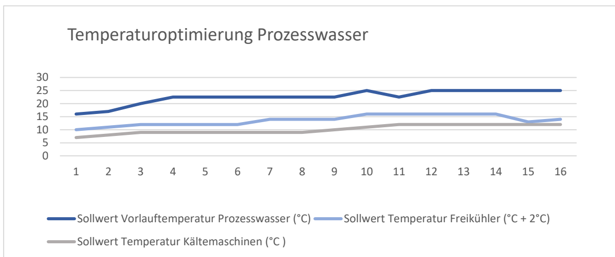
Abbildung 9: Temperaturoptimierung Prozesswasser
